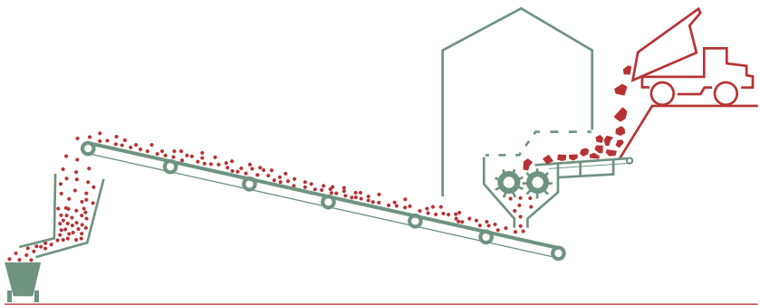
Brecheranlage mit Walzenbrecher
