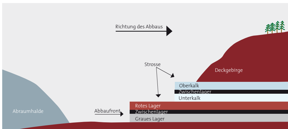
Abbauschema des Tagebaubetriebes
