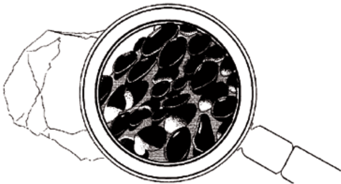
Die Ooiden kann man mit einer Handlupe untersuchen
